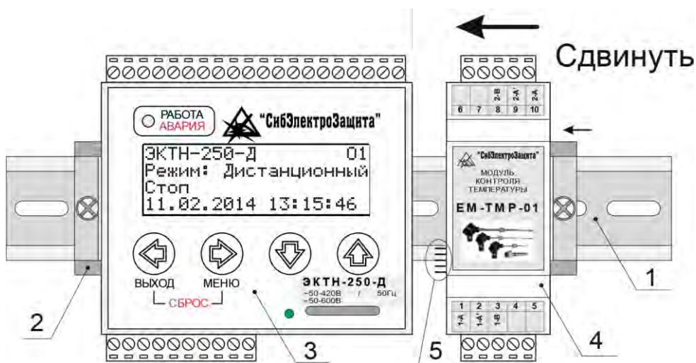
Рисунок 2 – установка внешнего модуля через разъем MD
