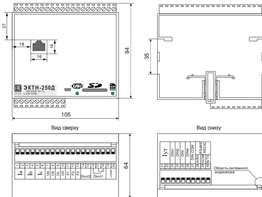
Рисунок 6 - Габаритные и установочные размеры базового модуля ЭКТН ВД.
