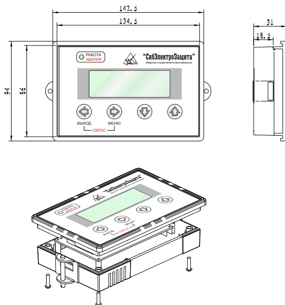
Рисунок 5 - Габаритные и установочные размеры выносного дисплея ЭКТН ВД.
