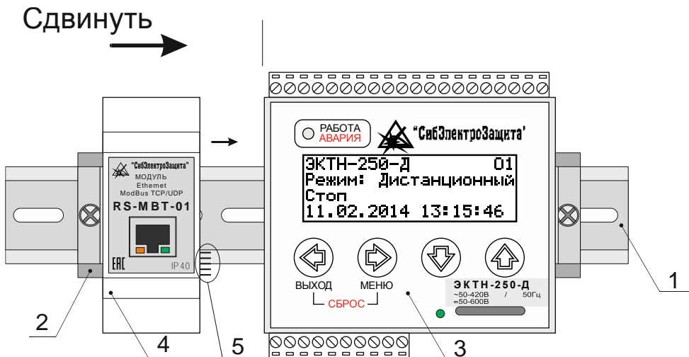
Рисунок 3 - Установка внешнего модуля через разъем MR
